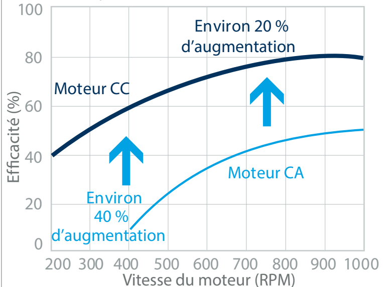
Efficacité du moteur CC* (comparaison avec un moteur CA conventionnel)
